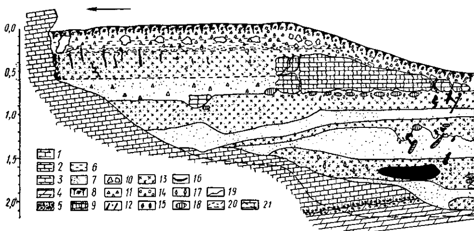
Рис. 6. Стратиграфія відкладів південної стінки розкопу стоянки Заскельне VI.
