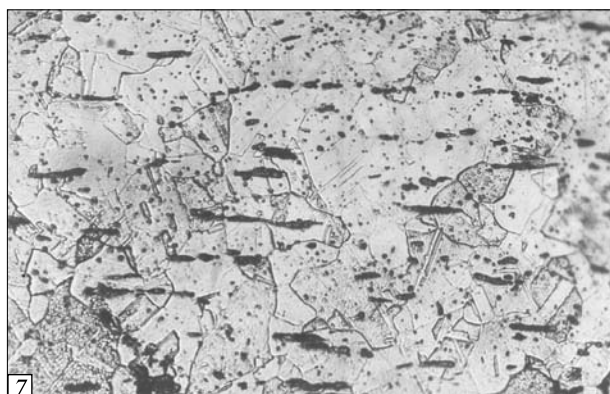
Рис. 2. Мікροструктури металу (зб. — збільшення): 1 — ан. 82, зб. 115; 2 — ан. 82, зб. 200; 3 — ан. 82, зб. 200; 4 — ан. 93, зб. 115; 5 — ан. 94, зб. 200; 6 — ан. 95, зб. 120; 7 — ан. 96, зб. 200
