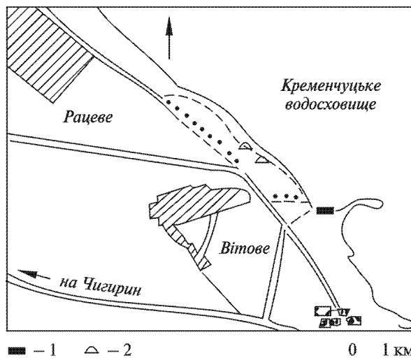
Рис. 1. Розташування поселення біля с. Вітове. Схематичний план: 1 — поселення; 2 — курган
