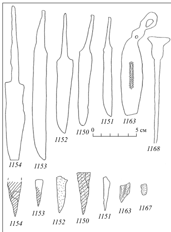
Рис. 1. Технологічні схеми залізних виробів із Витачева
