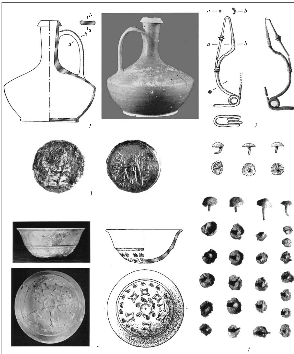
Рис. 6. Некрополь Богазкея. Кам'яна гробниця № 12, південний сектор, інвентар: 1 — червонолаковий горщик; 2 — залізна фібула; 3 — срібна монета Аріобазарна I (Кападокія); 4 — залізнi цвяхи (оббивка підшов сандалій) (Kühne 1969; Boehmer 1972); 5 — «мегарська» чашка
