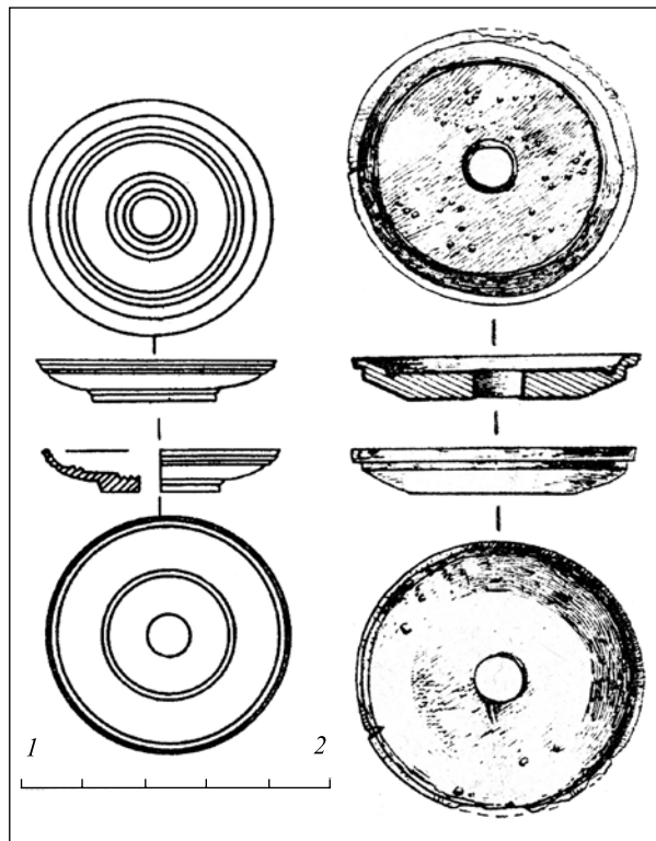
Рис. 4. Кістяні дископодібні насадки: 1 — Соболева Могила; 2 — Первомайка, кург. 2
