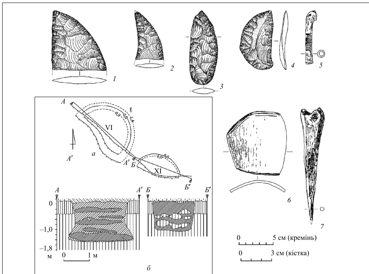
Рис. 6. Дубно-Волиця-2. Об'єкти VI і XI: 1—4 — вироби з кременю; 5, 7 — кістка. На врізці: а — плани; б — розрізи об'єктів по лініях А—А' і Б—Б' (умовні позначення див. на рис. 2)
