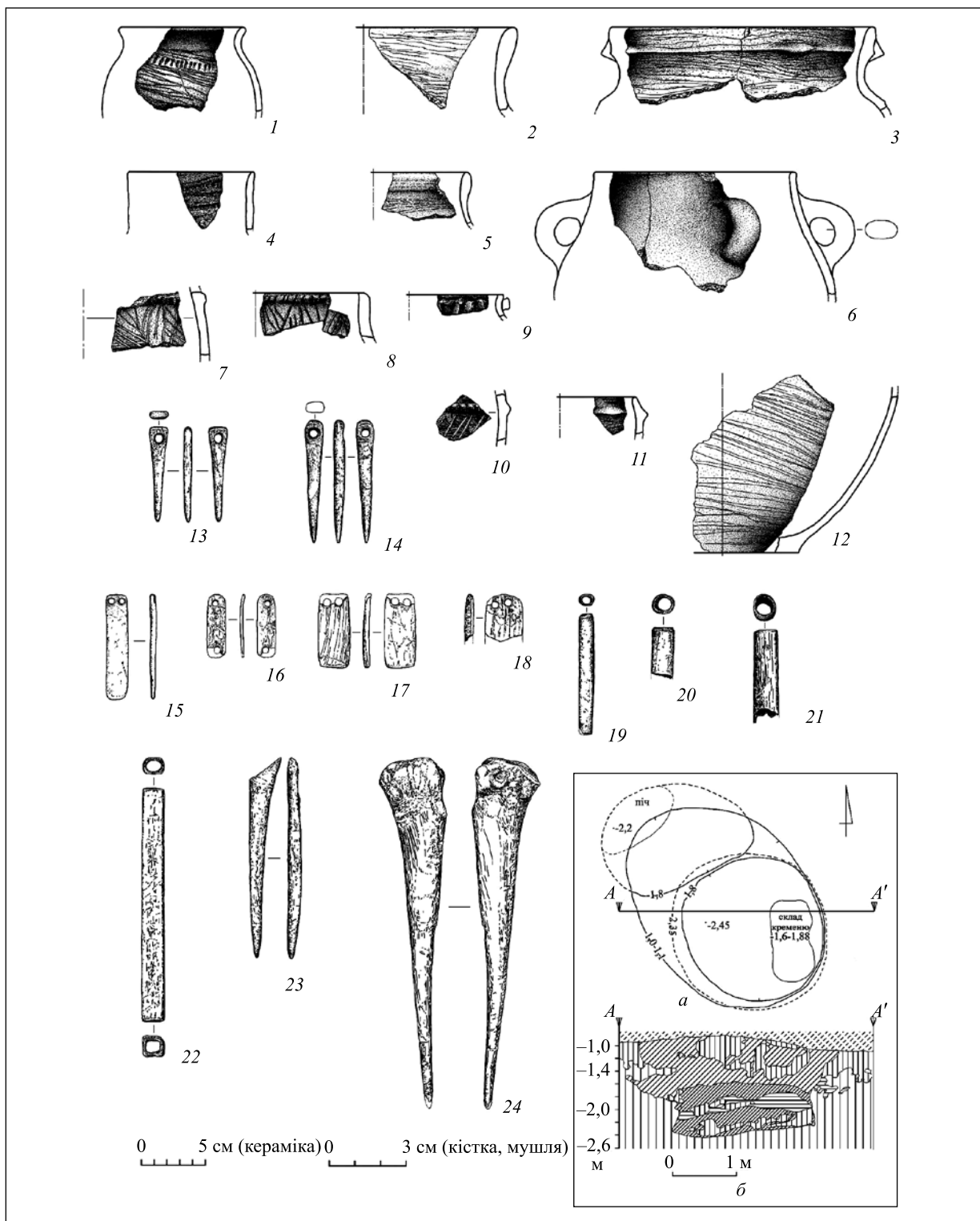
Рис. 10. Дубно-Волиця-2. Об'єкт XVI: 1—12 — кераміка; 13—24 — кістка, мушля. На врізці: а — план; б — розріз по лінії А—А' (умовні позначення див. на рис. 2)
