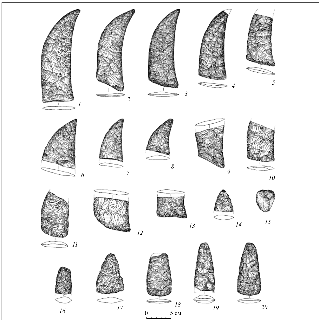
Рис. 9. Дубно-Волиця-2. Об'єкт XIII. Вироби з кременю
