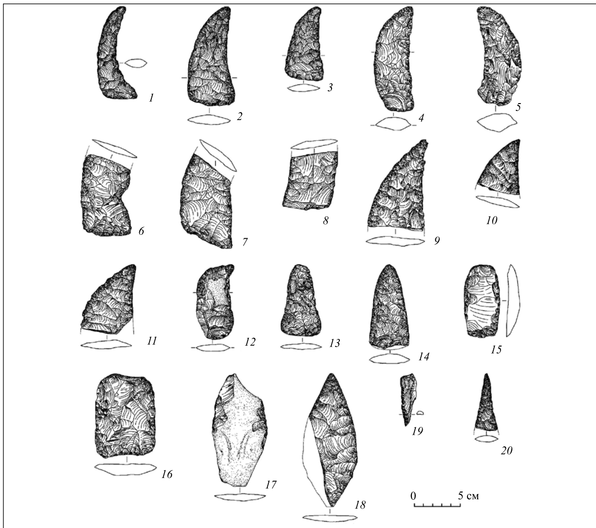
Рис. 11. Дубно-Волиця-2. Об'єкт XVI. Вироби з кременю
