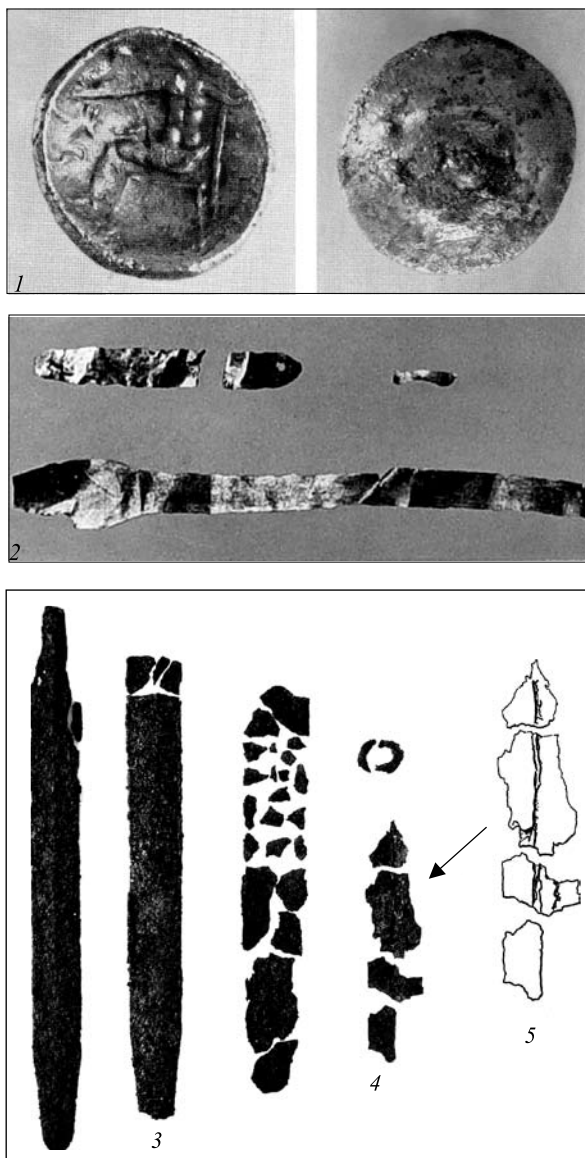
Рис. 5. Некрополь Богазкея. Інвентар кам'яної гробниці № 11, південний сектор (1 — срібна монета Брөгитара; 2 — деталі срібного вінка) і кам'яної гробниці № 3, південний сектор (3 — фрагменти залізного меча і залізних піхов; 4 — фрагменти залізного перся; 5 — фрагменти залізного наконечника списа) (Kühne 1969; Boehmer 1972)
