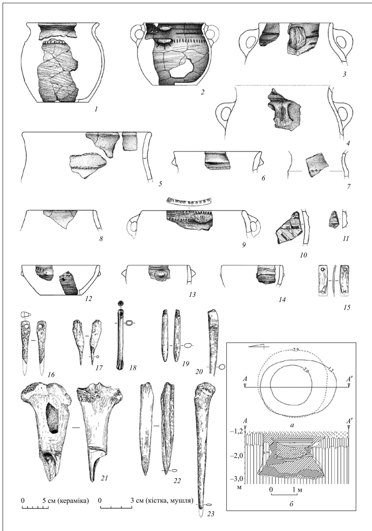
Рис. 8. Дубно-Волиця-2. Об'єкт XIII: 1—14 — кераміка; 15—23 — кістка, мушля. На врізці: а — план; б — розріз по лінії А—А' (умовні позначення див. на рис. 2)
