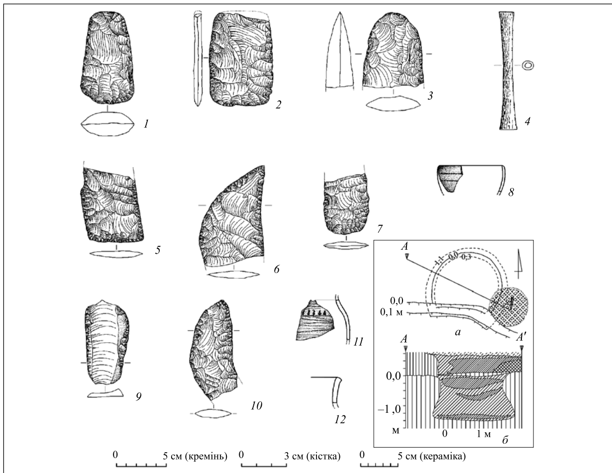
Рис. 4. Дубно-Волиця-2. Об'єкт III: 1—3, 5—7, 9, 10 — вироби з кременю; 4 — кістка; 8, 11, 12 — кераміка. На врізці: а — план; б — розріз по лінії А—А' (умовні позначення див. на рис. 2)
