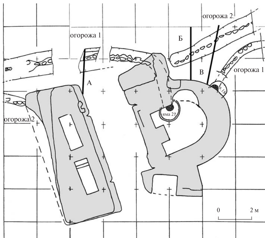
Рис. 2. Київ. План залишків огорожі 1 (перша чверть XII ст.), огорожі 2 (остання чверть XII ст.) і цегляної брами кінця XII ст. біля Михайлівського Золотоверхого собору
