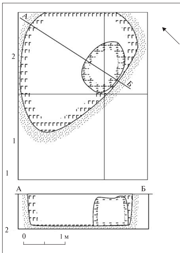
Рис. 1. Жидичин. План і перетин споруди 2
