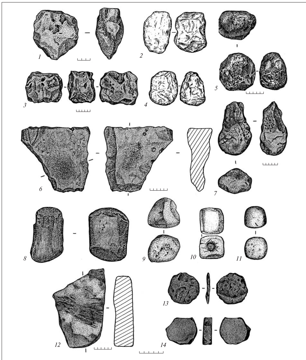
Рис. 2. Кам'яні знаряддя з техногенної ділянки копальні Червоне озеро І: 1 — мотика; 2—3 — прив'язні молоти; 4—5 — ручні молоти; 6 — рудодробильна (рудотерна) плита; 7 — товчак; 8 — чекан; 9—11 — рудодробильне (рудотерне) каміння; 12 — плита пісковика зі слідами ударів металевим знаряддям; 13—14 — диски
