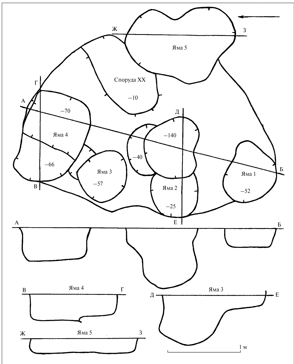
Рис. 2. Хрінники, уроч. Шанків Яр. План і розрізи споруди XX поморсько-кльошової культури
