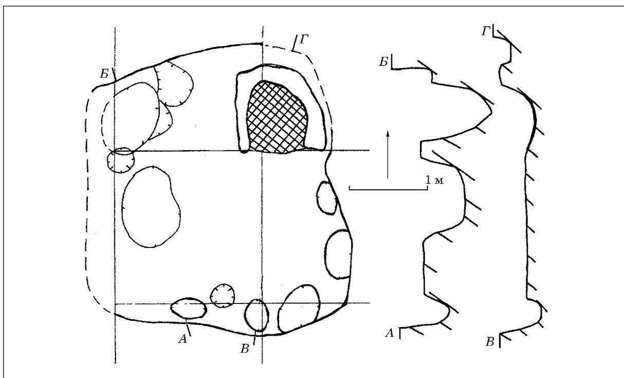
Рис. 57. План та розрізи житла 83
