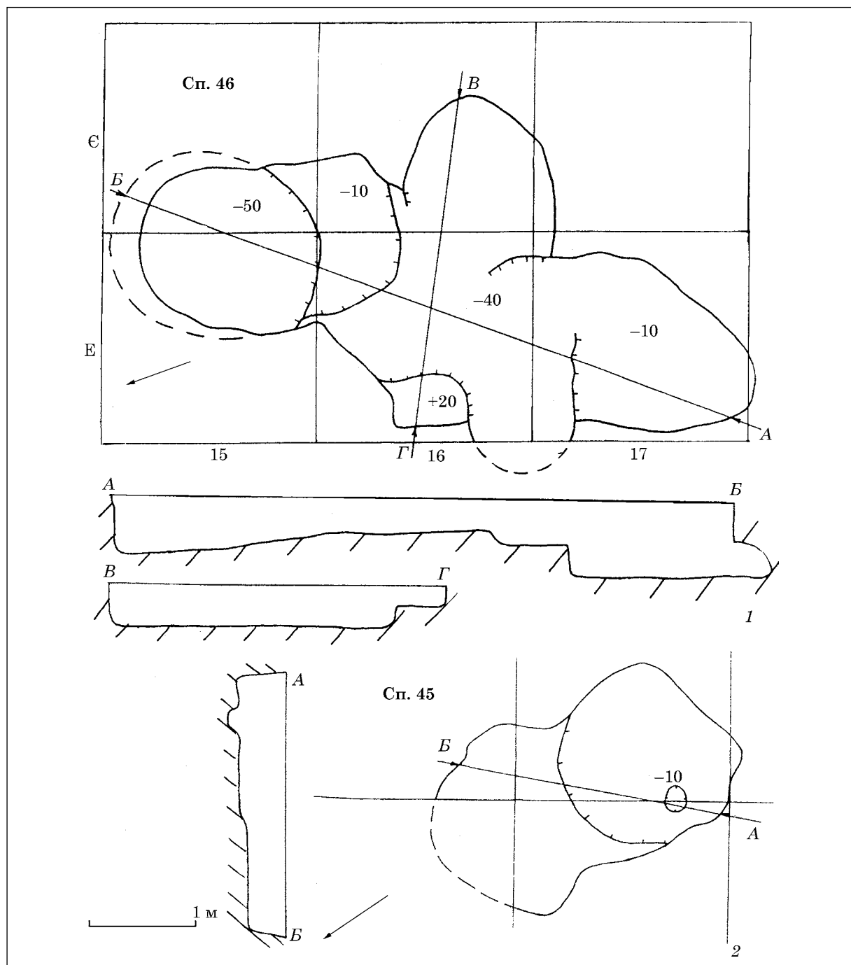
Рис. 6. Плани та розрізи споруд: 46 (1); 45 (2) (2003 р., р. XX)
