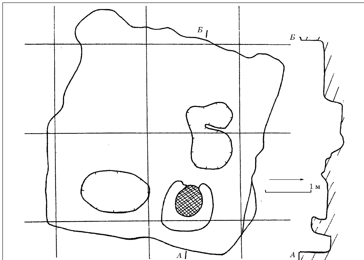
Рис. 71. План та розріз житла 94
