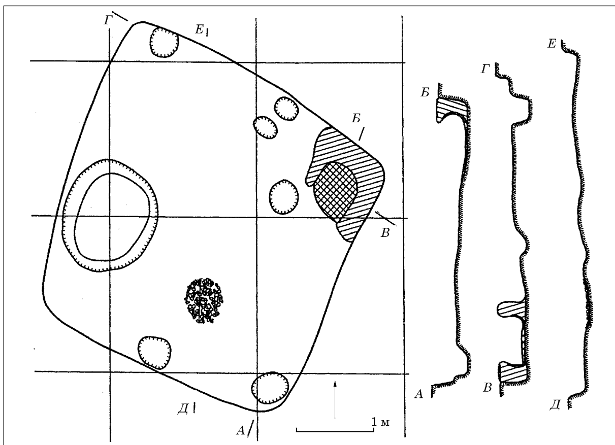
Рис. 65. План та розрізи житла 106
