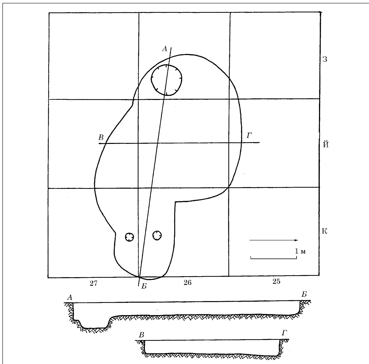
Рис. 24. План та розрізи житла 100
