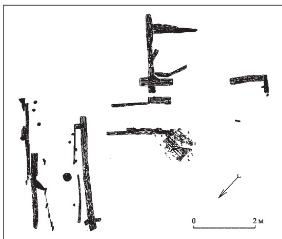
Рис. 25. План конструкцій XI ст. на Набережно-Хрещатицькій, 1-а
