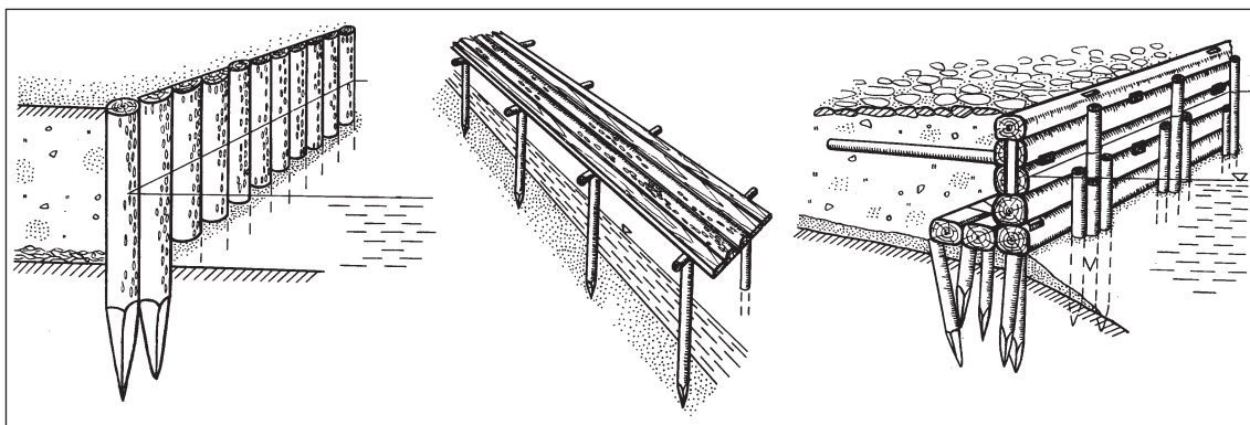
Рис. 28. Реконструкція берегових укріплень Ризької гавані у XII—XIV ст. (за А. Цауне)
