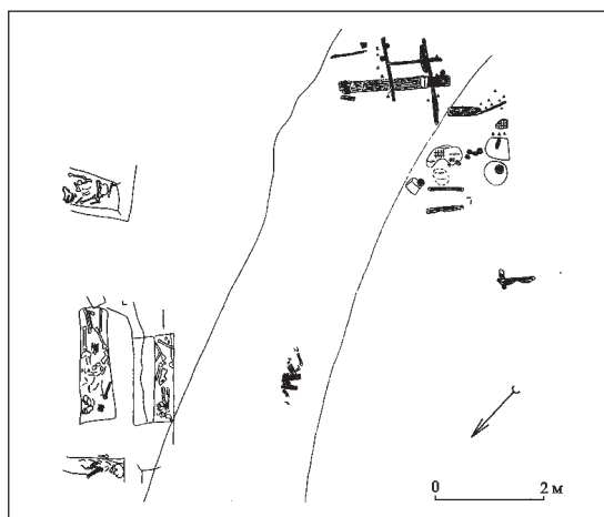
Рис. 26. Дренажний канал кінця XI ст. на Набережно-Хрещатицькій, 1-а
