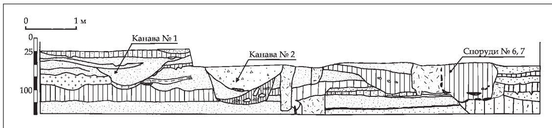
Рис. 36. Стратиграфічний розріз дороги з розкопу на вул. Григорія Сковороди, 14–16, 2006 р.
