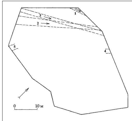
Рис. 17. План-схема напрямків водних потоків, зафіксованих на вул. Оболонській, 5
