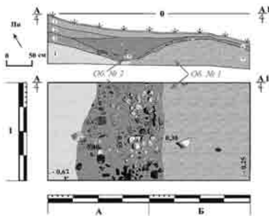
Рис. 2. Траншея ІІ (планіграфія та стратиграфія нашарувань північної стінки): 1 – гумусоно-аккумулятивний г-т, 2 – елювіальний г-т, 3 – ілювіальний г-т, 4 – вапнякова порода, 5 – заповнення об. № 2, 6 – чорні гумусовані суглинки (ілювіальний г-т ?), 7 – перевідкладений г-т вапняку
