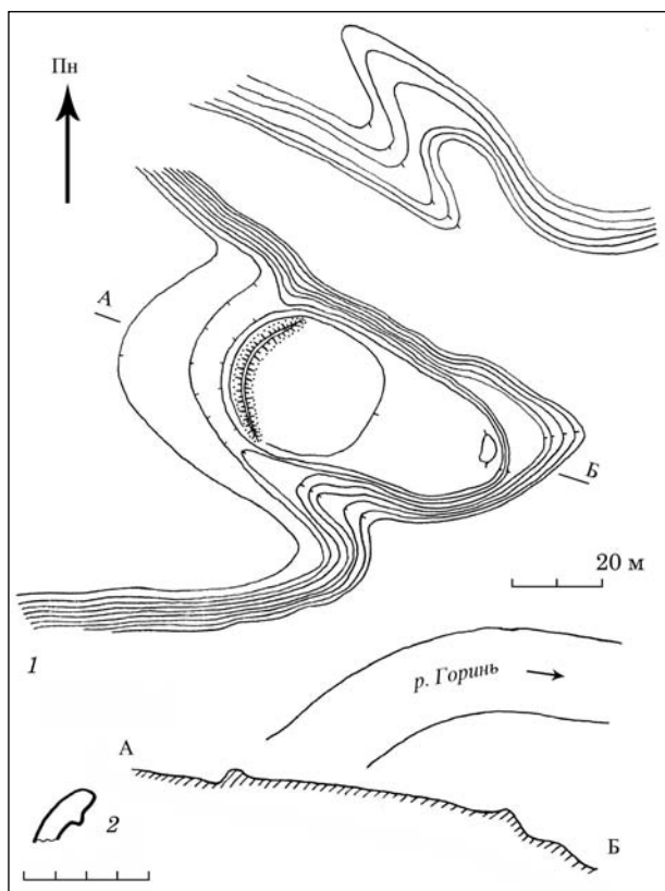
Рис. 3. Городище біля с. Бечаль: 1 – план городища; 2 – профіль в'янця гончарного горщика
