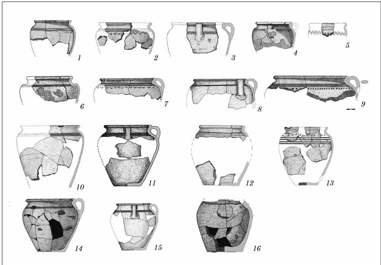
Рис. 9. Форми кухонних горщиків з даного поселення
