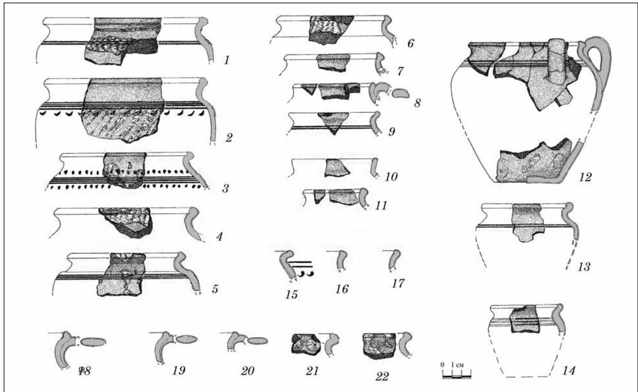
Рис. 1. Полів'яні горщики з поселення Ходосівка-Рославське
