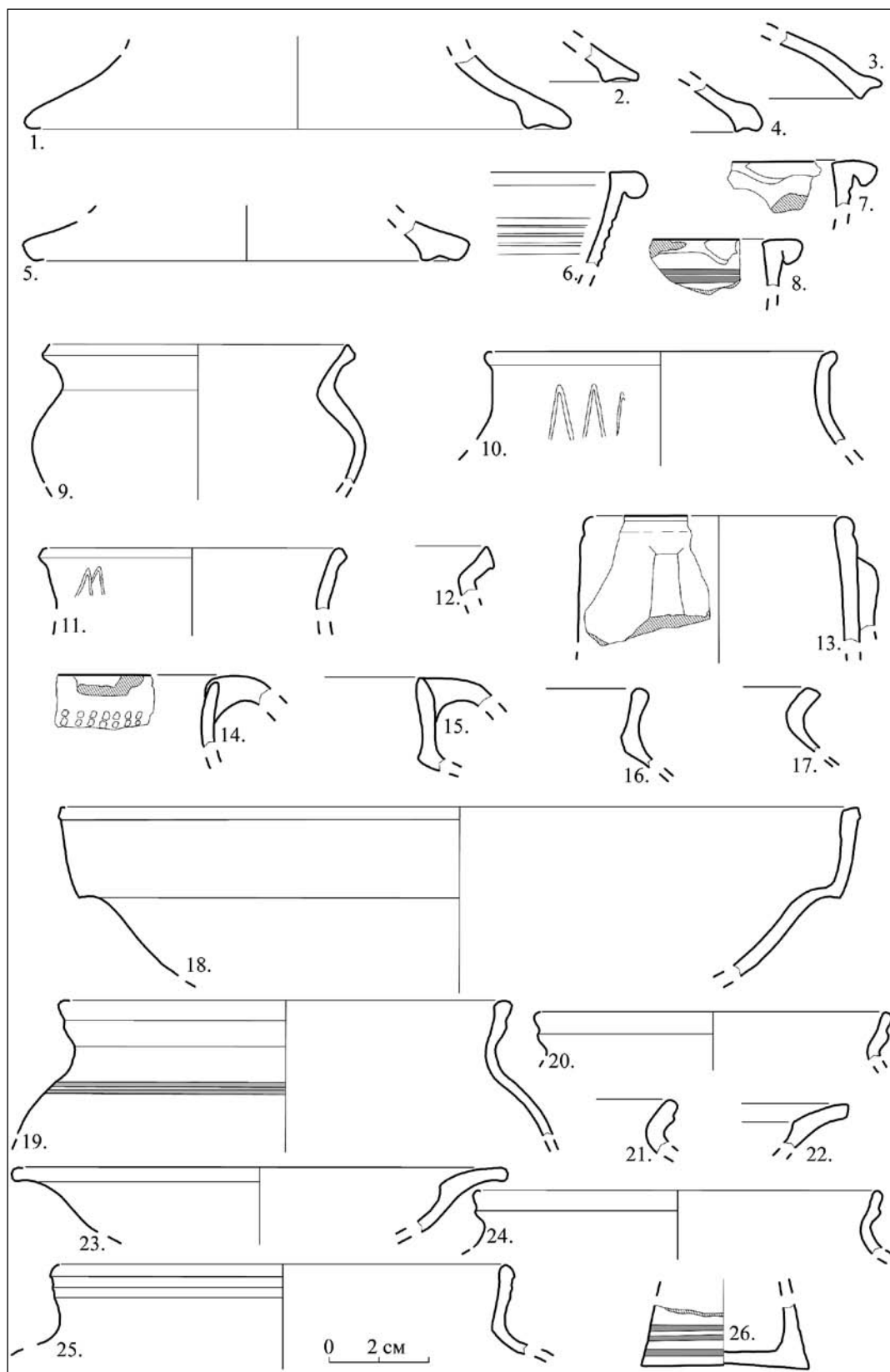
Рис. 7. Знахідки із культурного шару розкопу № 1 біля Свято Миколаївської церкви. 1–8 – гончарні вінця покритшок та макітр XVI–XVII ст.; 9–26 – гончарні посудини XVII–XVIII ст.
