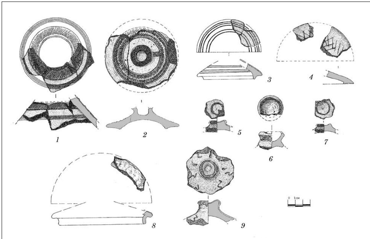
Рис. 4. Полив'яні (1, 3, 5, 7, 8, 9) та неполив'яні (2, 4, 6) кришки з поселення в урочищі Рославське
