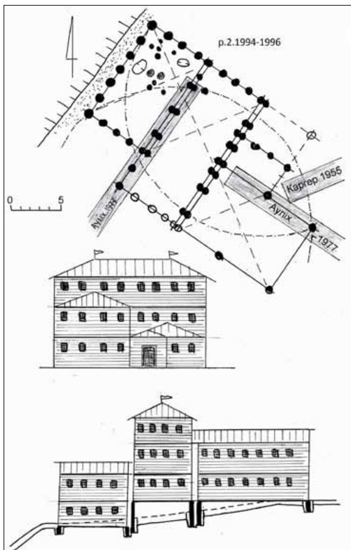
Рис. 4. Крилоське городище. Княжий двір. Західний палацовий комплекс
