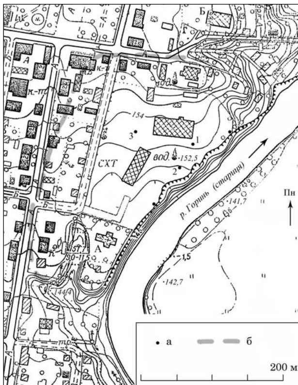
Рис. 10. План центральної частини м. Дубровиця. Буквами позначені: А – Миколаївська церква; Б – костел Іоанна Хрестителя. Умовні позначення: а – археологічні шурфи та зачистки берегового урвища; б – вірогідна лінія середньовічних укріплень
