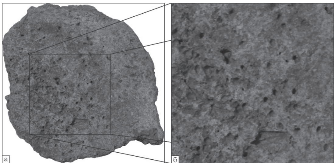
Рис. 8. Мала Снітинка, денце з великою кількістю відбитків зернівок проса ( Panicum miliaceum ) й двома — жита ( Secale cereale ): а — натуральна величина; б — подвійне збільшення (фото М. С. Сергеевої)
