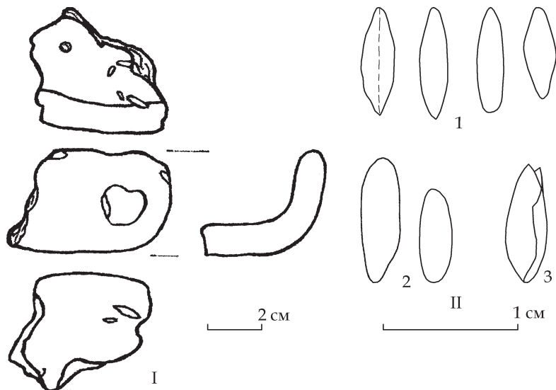
Рис. 7. Лтава, розкоп 4 1997 р.: I – фрагмент ліпної сковорідки № 201 (прорисовка К. М. Мироненка); II – відбитки зернівок культурних рослин на ньому: 1 – жито ( Secale cereale ); 2 – овес ( Avena sativa ); 3 – ячмін півлчасний ( Hordeum vulgare )
