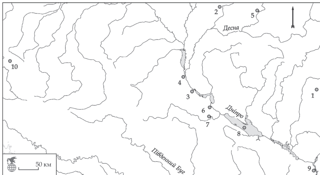
Рис. 11. Карта поширення знахідок шаблонів ювелірних виробів: 1 — Козіївка / Нова Одеса; 2 — Мощенки; 3 — Девіча Гора; 4 — Київ; 5 — Дегтярівка; 6 — Канів, в т. я. Княжа Гора; 7 — Сахнівка; 8 — Середнє Подніпров'я; 9 — Дніпровське Надпоріжжя; 10 — Зимне
