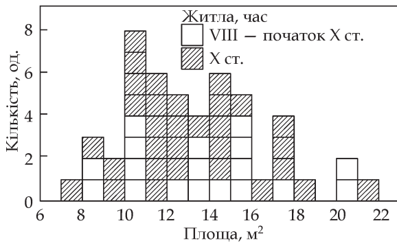
Рис. 2. Гістограма розподілу за площею жител райковоцької культури в басейні р. Горині
