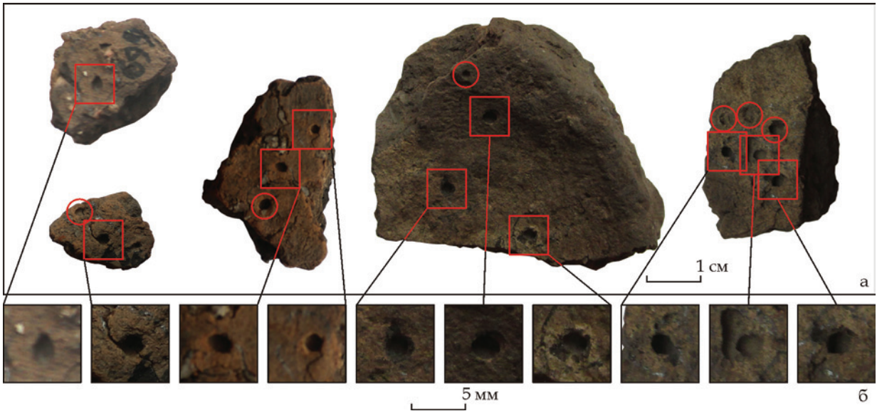
Рис. 4. Борисковичі, житло 1, фрагменти ліпної кераміки другої—третьої чверті I тис. н. е. з відбитками зернівок проса ( Panicum miliaceum ) (фото А. Ф. Касюк)
