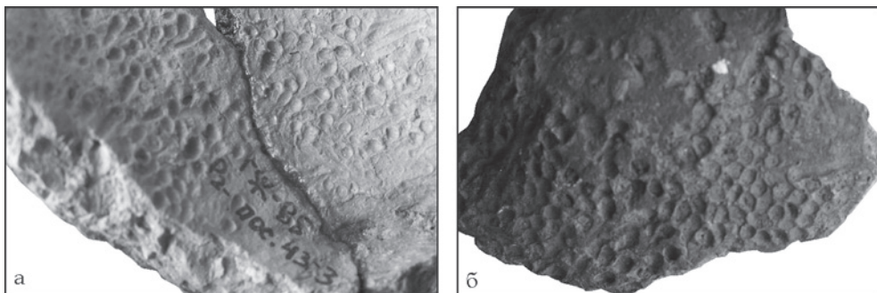
Рис. 12. Животинне городище, будівля 43, фрагменти горщика, суцільно вкритого відбитками зернівок проса ( Panicum miliaceum ): а — внутрішня сторона; б — зовнішня сторона (фото В. М. Ковалевського)
