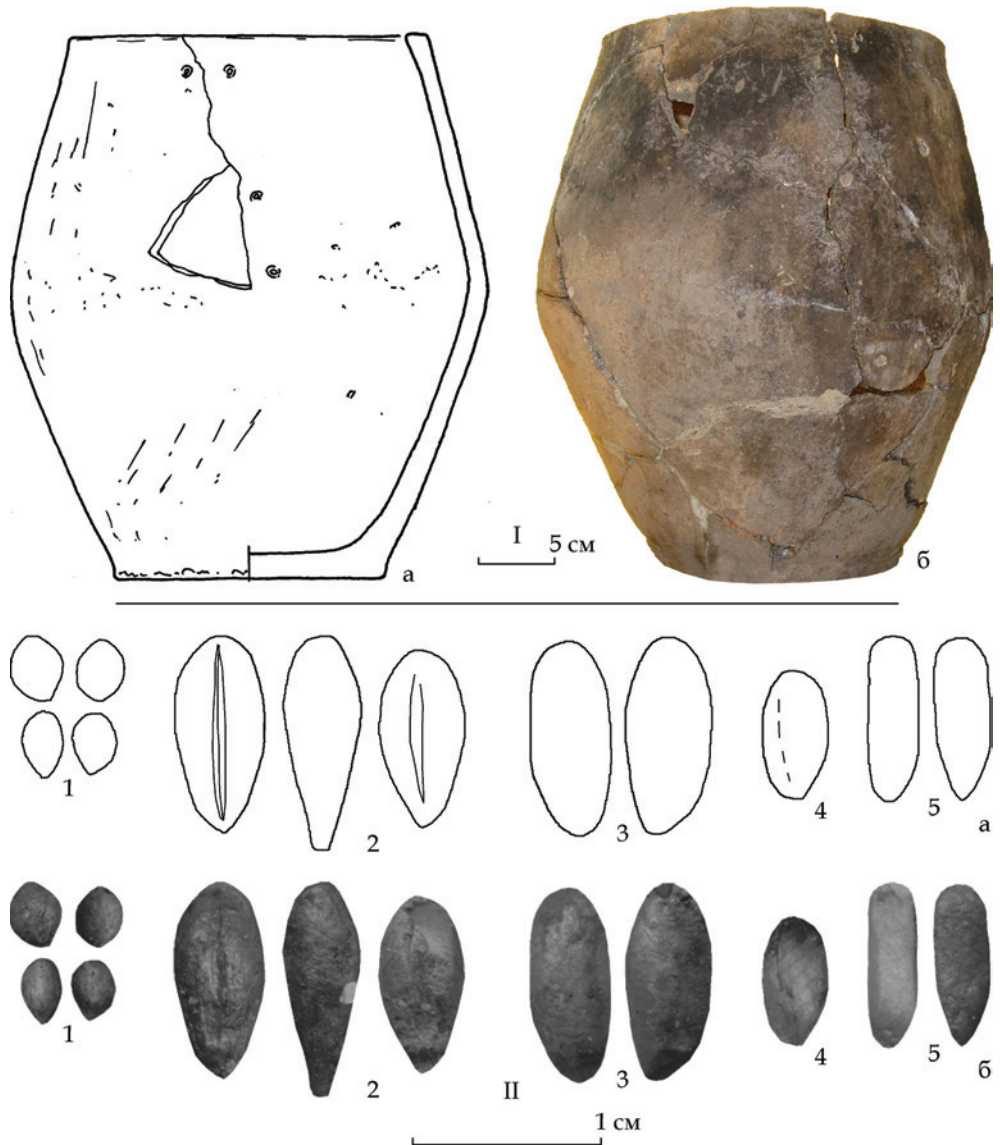
Рис. 2. Дмитрівка III: I — реконструйований праслов'янський зерновик (автор Ю. Ю. Башкатов); II — відбитки зернівок культурних рослин на ньому: 1 — просо ( Panicum miliaceum ); 2 — ячмінь півчастий ( Hordeum vulgare ); 3 — пшениця двозернянка ( Triticum dicoccon ); 4 — пшениця одностернянка ( Triticum monosocum ); 5 — жито ( Secale cereale ); а — прорисовки; б — фото
